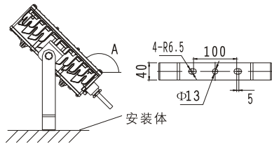
座式 (安装角度 0^{\circ} < A < 135^{\circ} )
