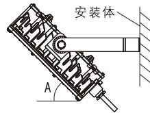
侧壁式 (安装角度 0^{\circ} < A < 90^{\circ} )
